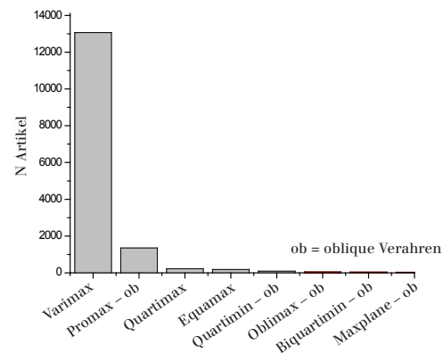
Abbildung 2: Anzahl von Artikeln, in denen auf Faktorenrotation der Einfachstruktur verwiesen wird. Ergebnis einer Internet-Suche nach Rotationsbezeichnungen in SCIENCE DIRECT (Elsevier, 2008)
