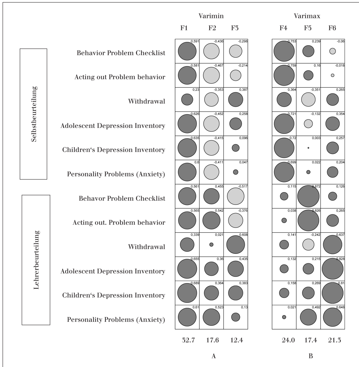
Abbildung 14: Varimin-(A) und Varimaxlösung (B) der Matson & Nieminen-Daten (1987)
